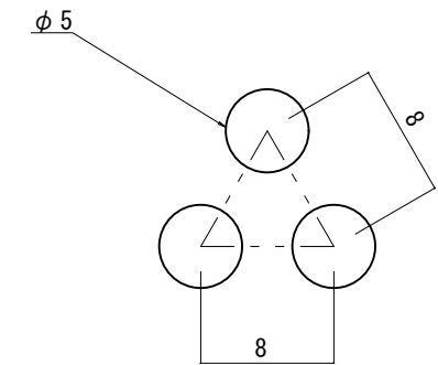
パンチングメタル寸法図
