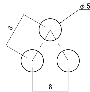
パンチング寸法図 S=2/1
